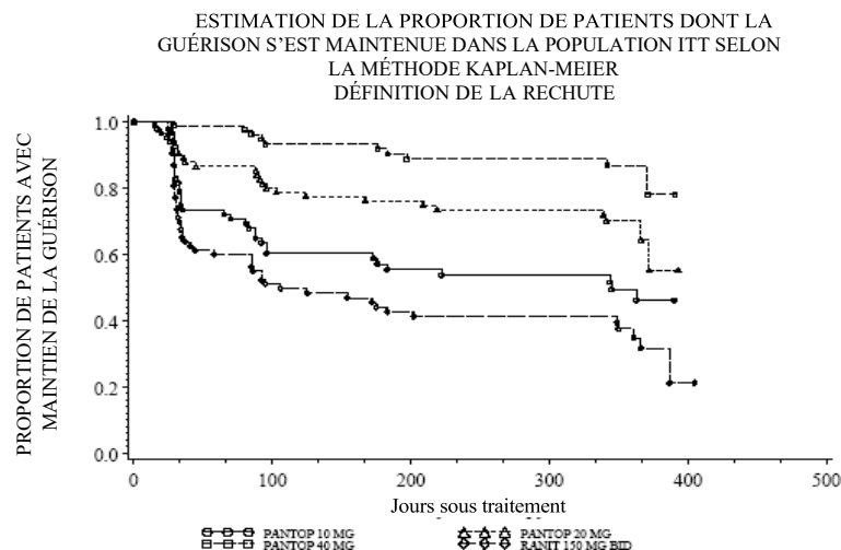
Figure 1 – Courbe de l'analyse de Kaplan-Meier; 3001A1-302-US
